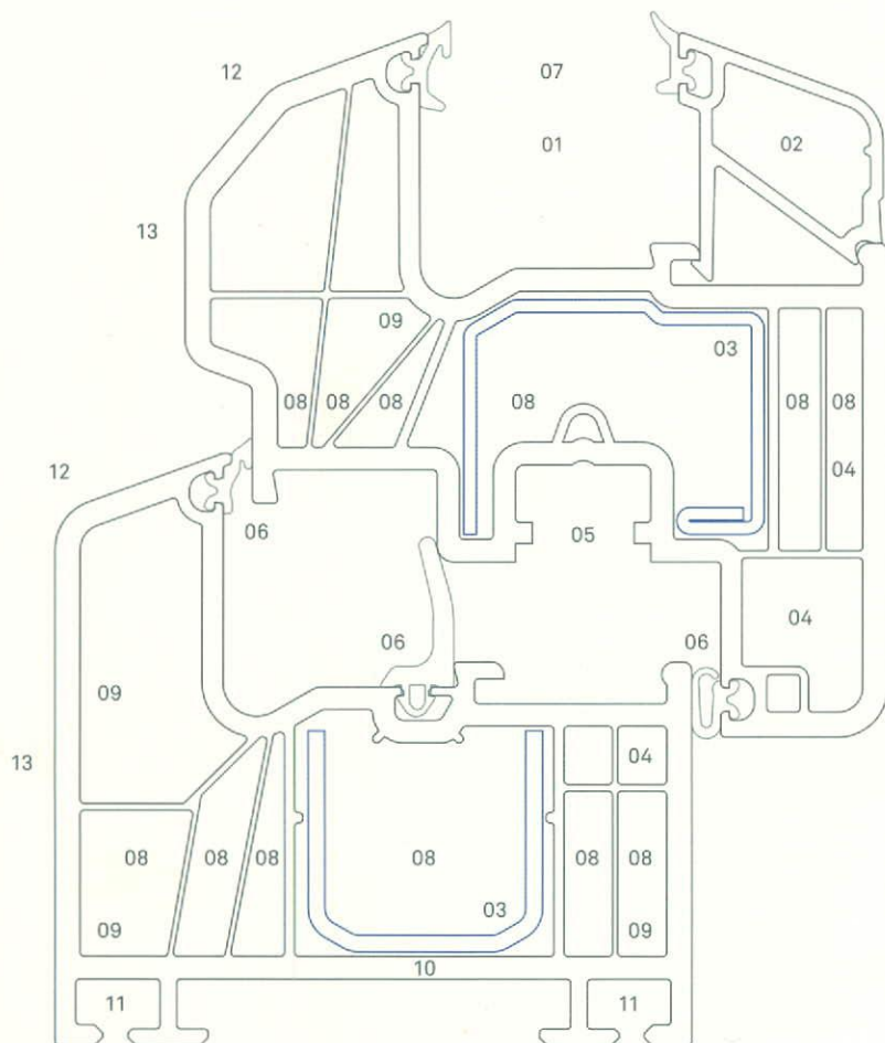
Szögletes vízvetőszárnyas kialakítású Prestige / középtömítés (MD) Ábra: 1:1
