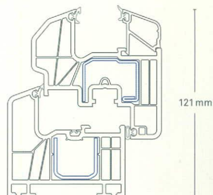
Ütközőtömítés (AD) Ábra: 1:25
